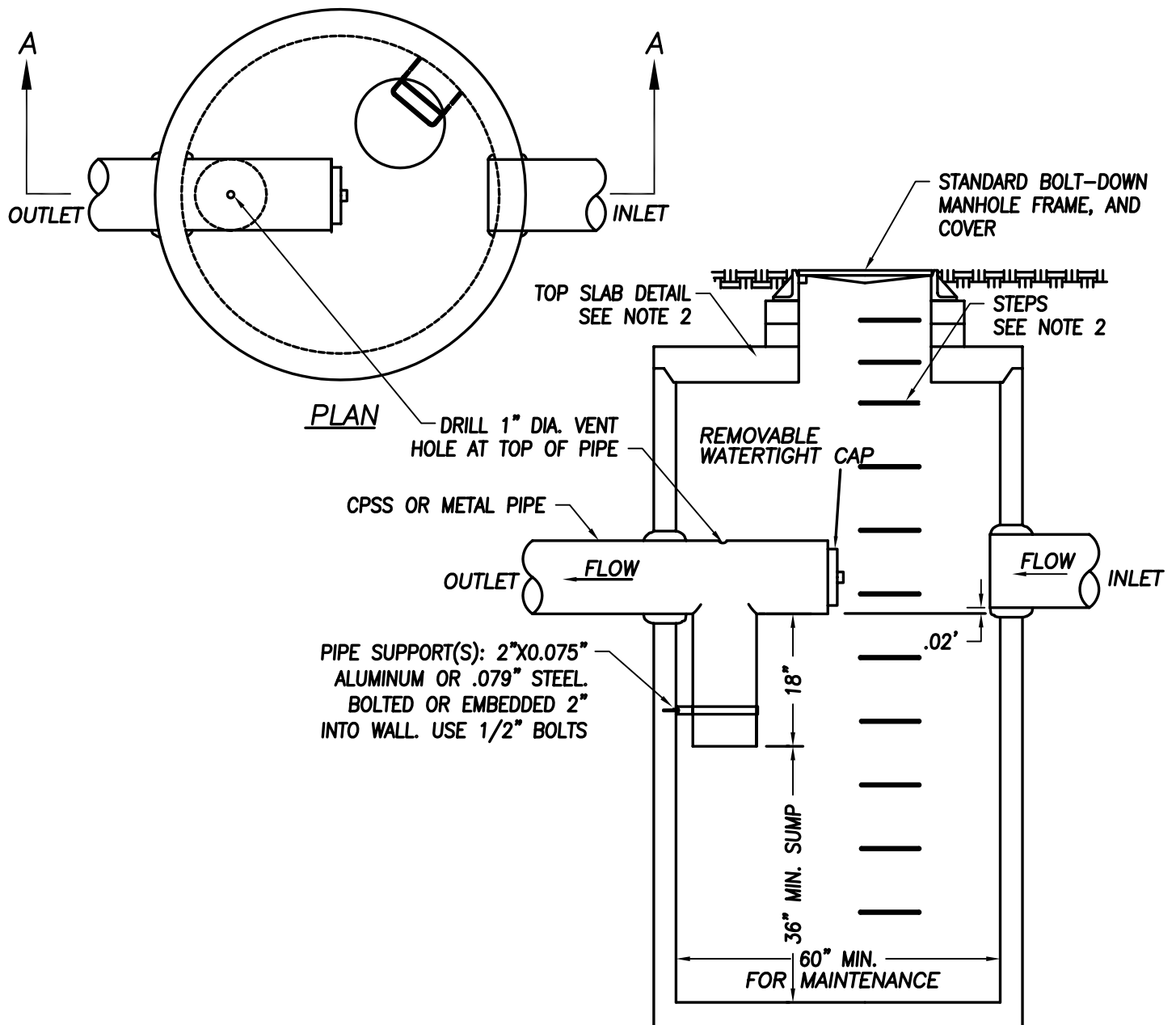
SECTION A-A
