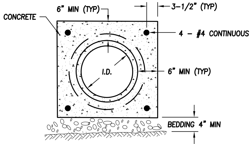
VIEW A-A
